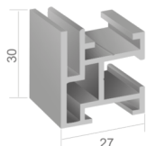
720426 - Miniframe 30mm
